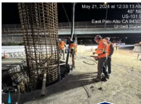
Concrete Pour
