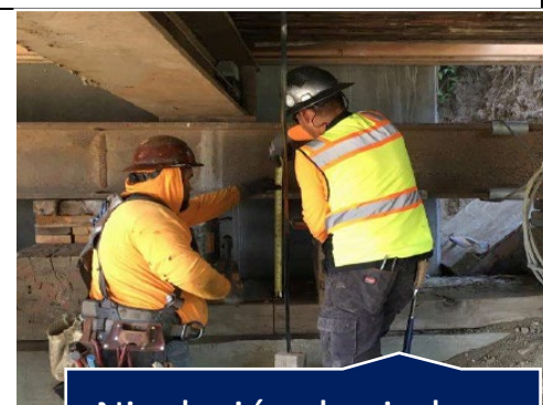
Nivelación de cimbras dobladas
